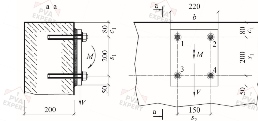
Рисунок 3.1 – Пример 3. Схема анкерного крепления
