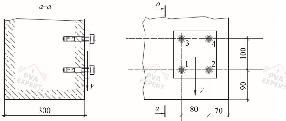
Рисунок 2.1 – Пример 2. Схема анкерного крепления.
