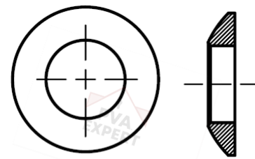
Kugelscheibe
